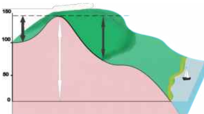
13. Баландии нисбӣ (тирчаи сиёҳ) ва мутлақӣ (тирчаи сафед) теппа
