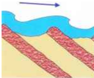
61. Нақшаи остонаи дарё
