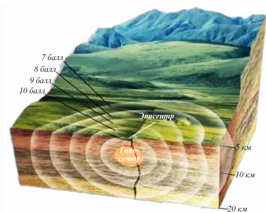
32. Манбаъ, марказ ва паҳншавии мавҷҳои zilzila
