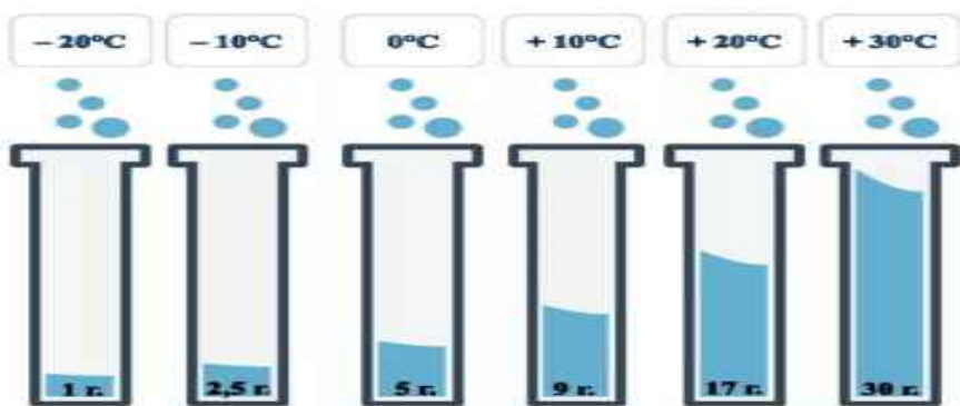
73. Вобастагии миқдори бухори об дар ҳавои сер аз ҳарорати он
