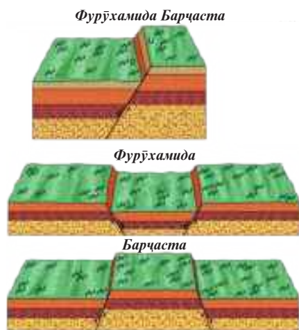
30. Фурӯҳамида ва барҷаста- ғиҳои рӯйи Замин
