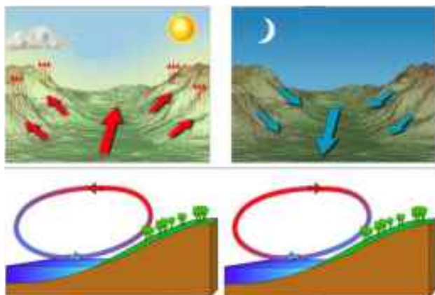
70. Тағйирёбии самти бод дар давоми шабонарӯз
